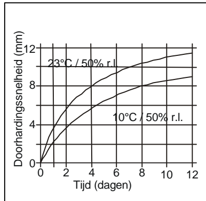
Schema 1: Uithardingstijd voor Sikaflex®-290 DC en Sikaflex®-290 DC SL (VP)
