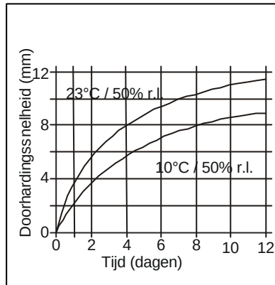
Schema 1: Uithardingstijd voor Sikaflex®-291
