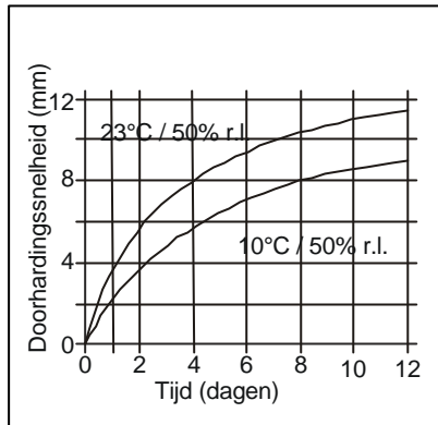
Schema 1: Uithardingsstijd voor Sikaflex®-292
