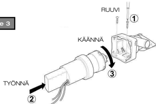
Kuva 2- Huom! Älä ruuvaa pumpua suoraan veneen pohjaan.
