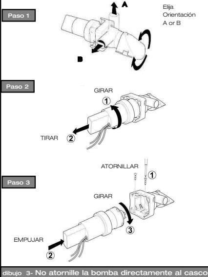
dibujo 3- No atornillar la bomba directamente al casco
